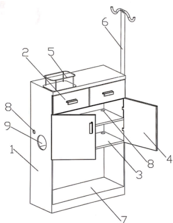
图 1 床头顶柜的设计
